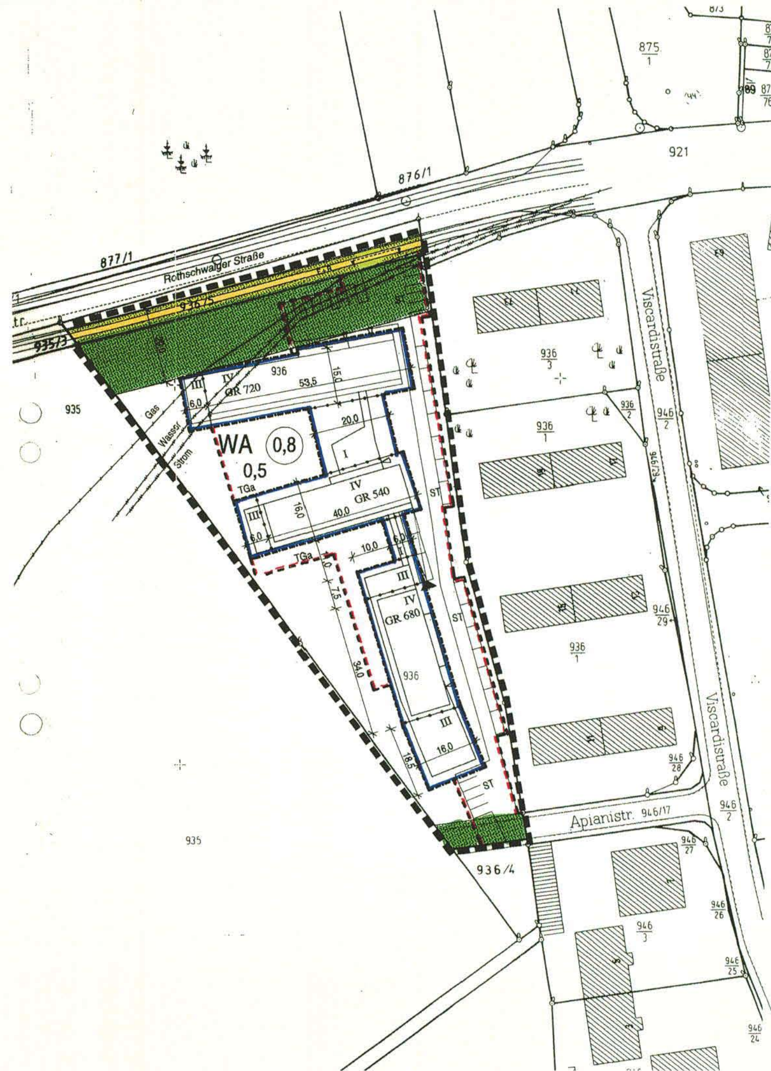
Planteil Bebauungsplan
